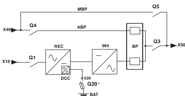
ALIMENTATION SÉPARÉE REDRESSEUR ET BY-PASS
