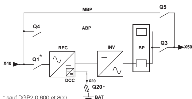
ALIMENTATION COMMUNE REDRESSEUR ET BY-PASS
