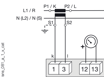
SC 1 : transducteur de courant autoalimenté (CSA-A)
