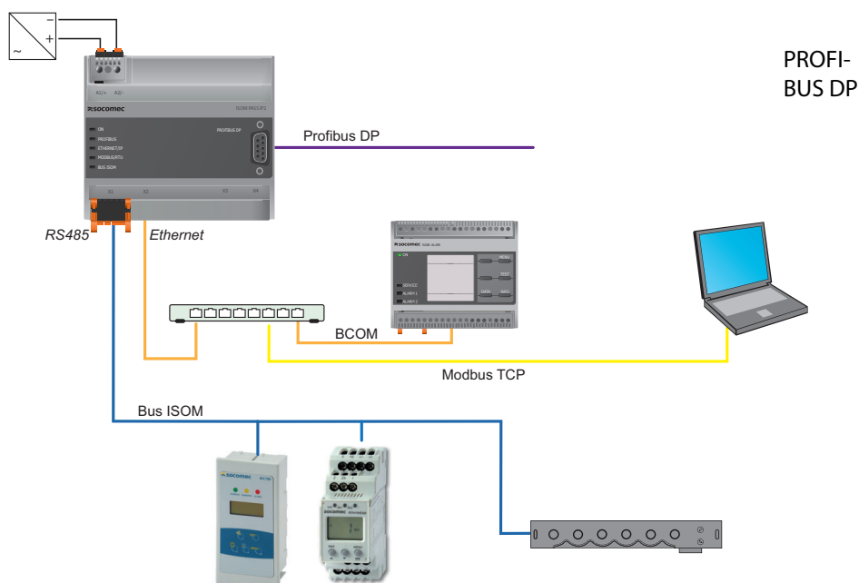
Fig. 4.2: Schéma de branchement ISOM PASS IP2
