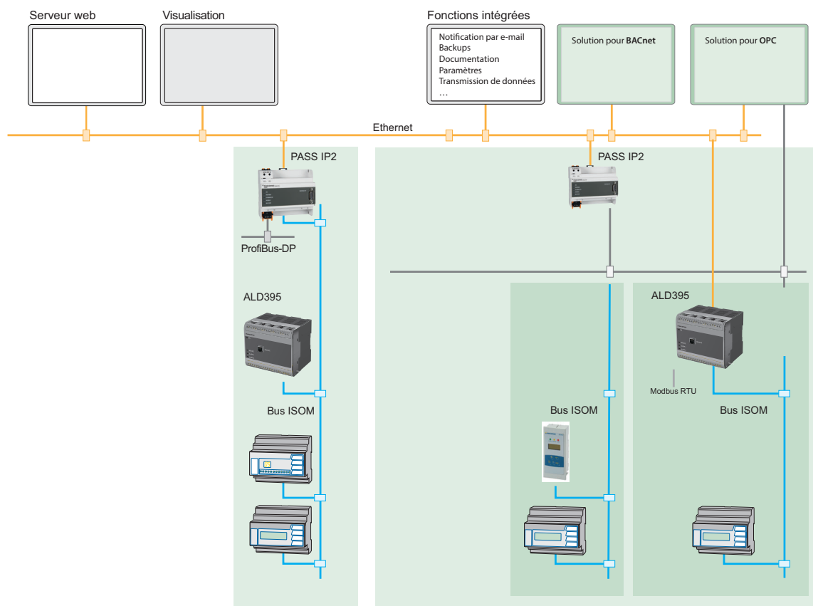
Fig. 3.1: Schéma de principe
