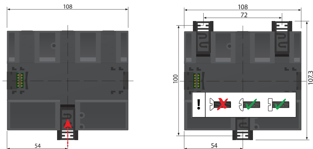
Fig. 4.1: Montage rail profilé, fixation par vis
