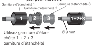
Fig. B Cable diameter 9 mm p.e. pour M25x1,5
