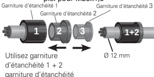
Fig. C Cable diameter 12 mm p.e. pour M25x1,5
