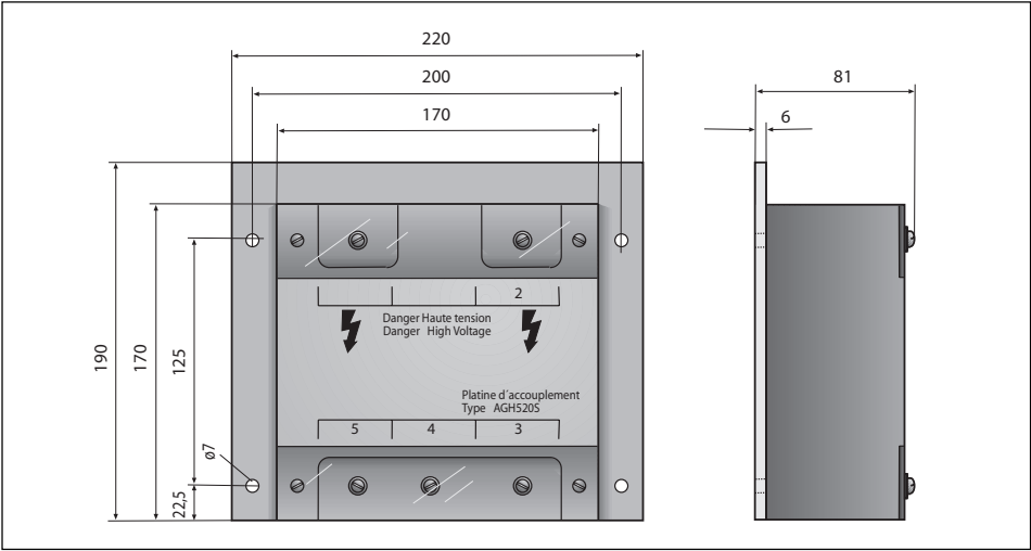
Encombrement Note
